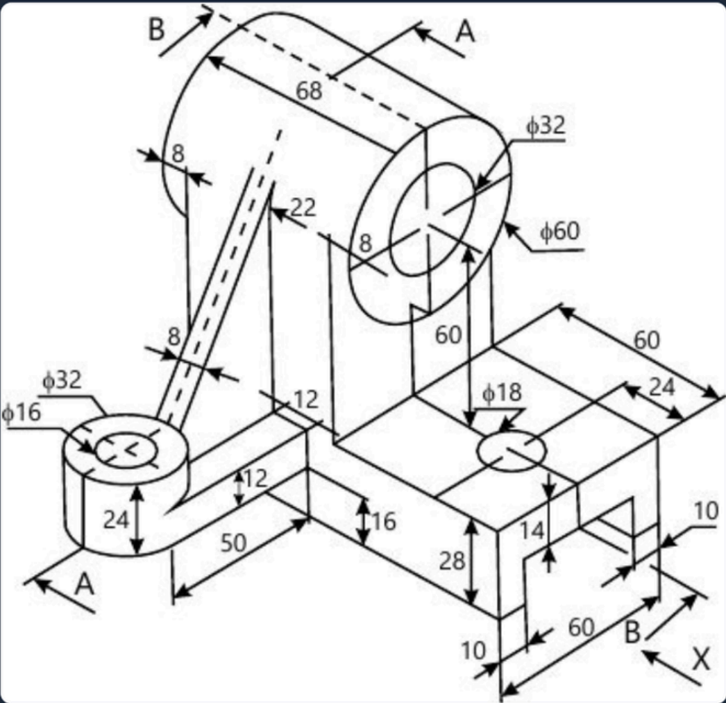
Suporte XYZ
